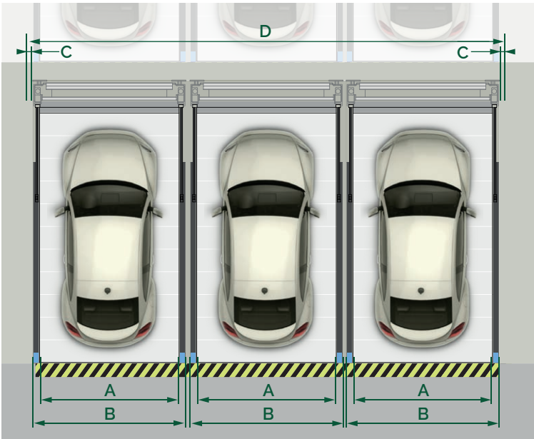
Jedes Segmentraster erfordert eine Zufahrt (Ein-/Ausfahrt).
