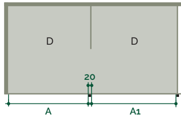
D = Doppelanlage für je 4 Pkw
